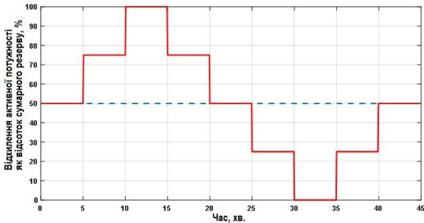
Рисунок 7. Сигнал АРП для перевірки петлі гістерезису аРВЧ як відсоток від повної резервної потужності одиниці надання ДП.
